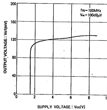
Fig.11 出力電圧 1 - 電源電圧特性
