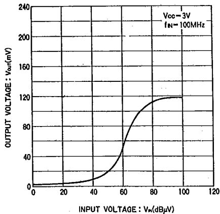
Fig.4 出力電圧-入力電圧特性
