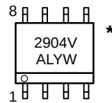
SO-8 VD SUFFIX CASE 751
