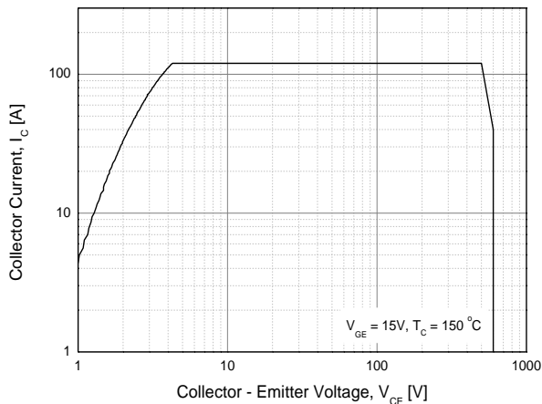
Fig. 15 RBSOA
